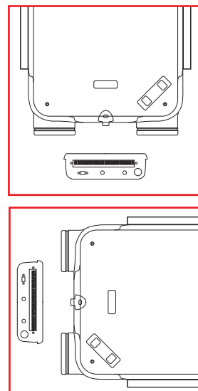
NESPRÁVNÉ instalace
